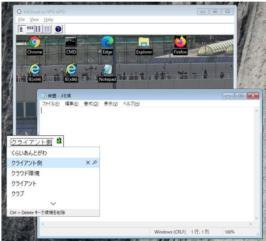
クライアント側 IME の実行例（未確定の文字を表示するウインドウを左上から移動）
